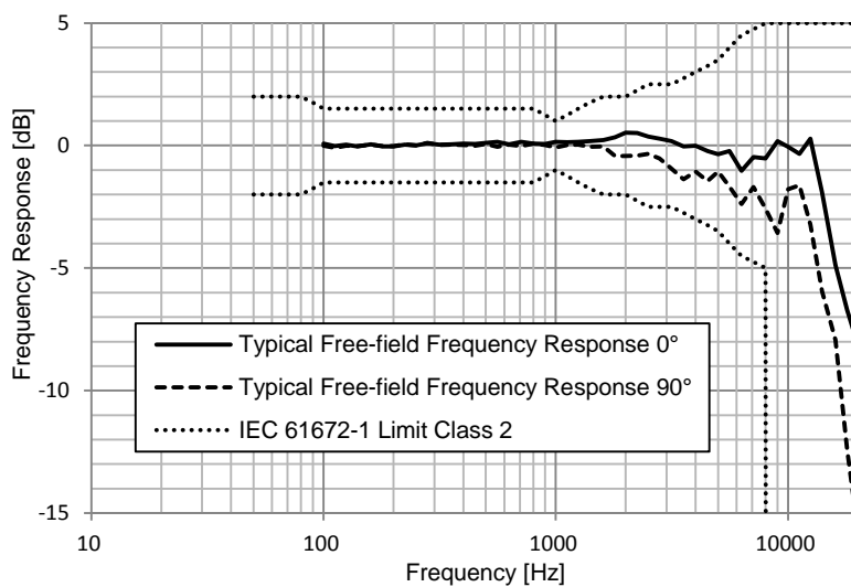
OM225 典型 0 度和 90 度入射自由场频率响应
